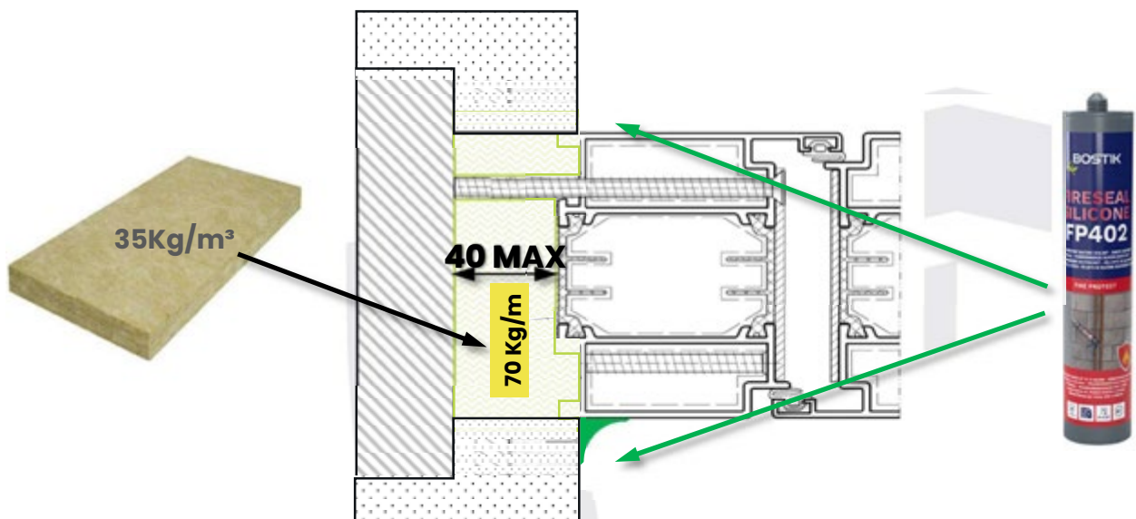
KOMBINATION STEINWOLLE/SILIKON
