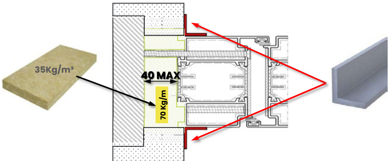
KOMBINATION STEINWOLLE/ALUMINIUMWINKEL
