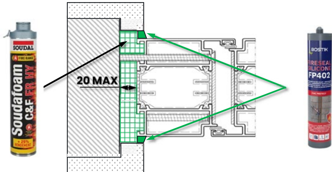
KOMBINATION PU-SCHAUM/BRANDSCHUTZSILIKON
